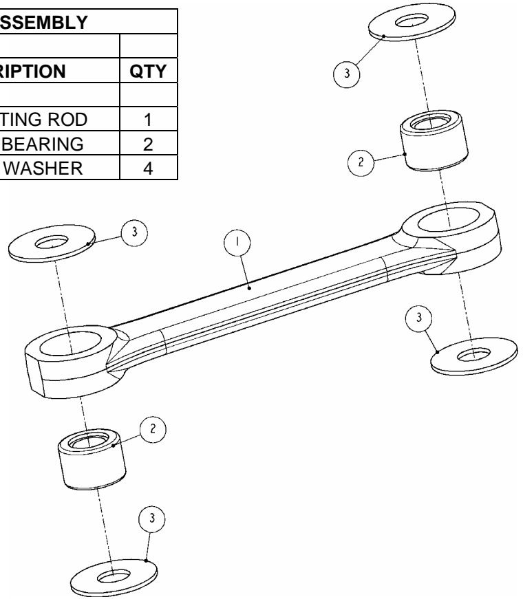
Figure 8 1901100: CON ROD
